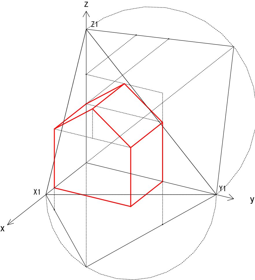
(1) 軸測投象
