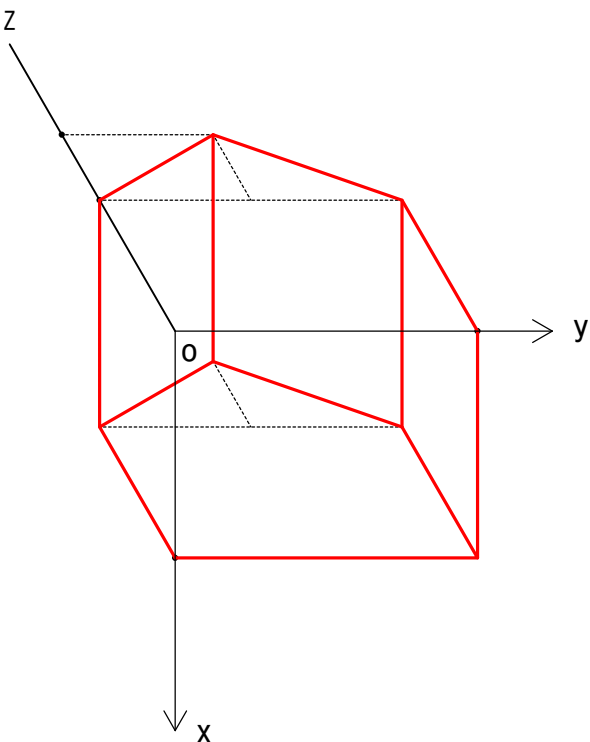
(3) ミリタリ投象 ( \delta=60^\circ \mu=2/3 )
