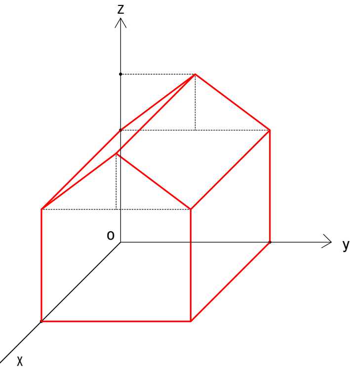
(2) カバリエ投象 ( \delta=45^\circ \mu=1 )
